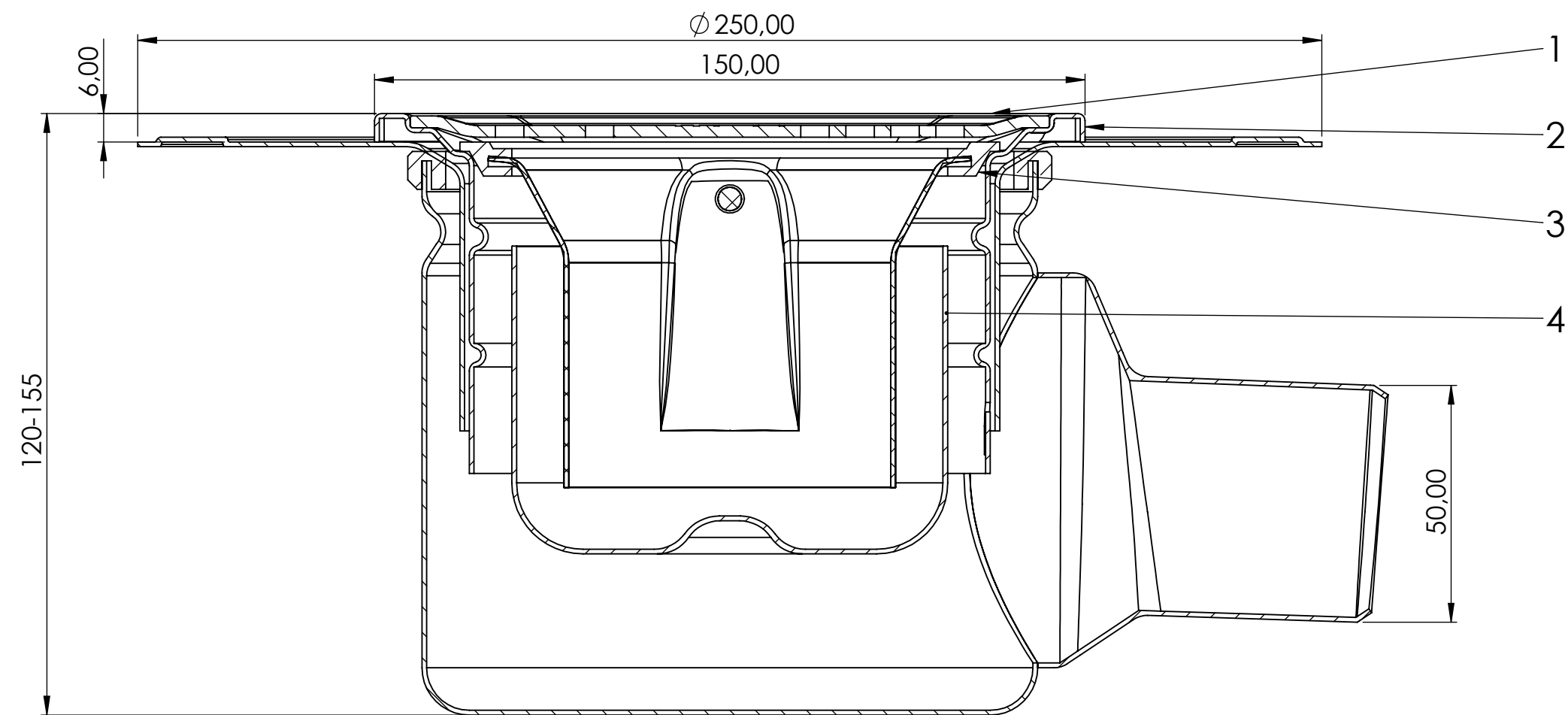
SECTION A-A
